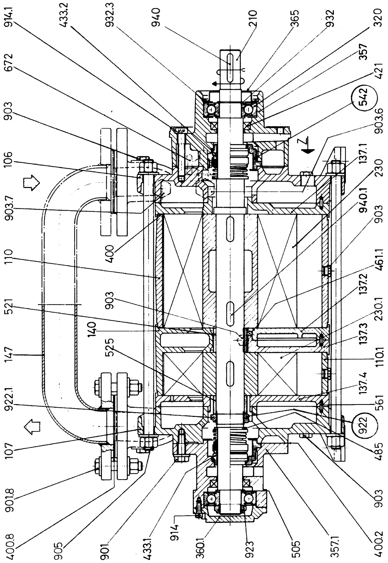
TRHC 40-140 & 190
