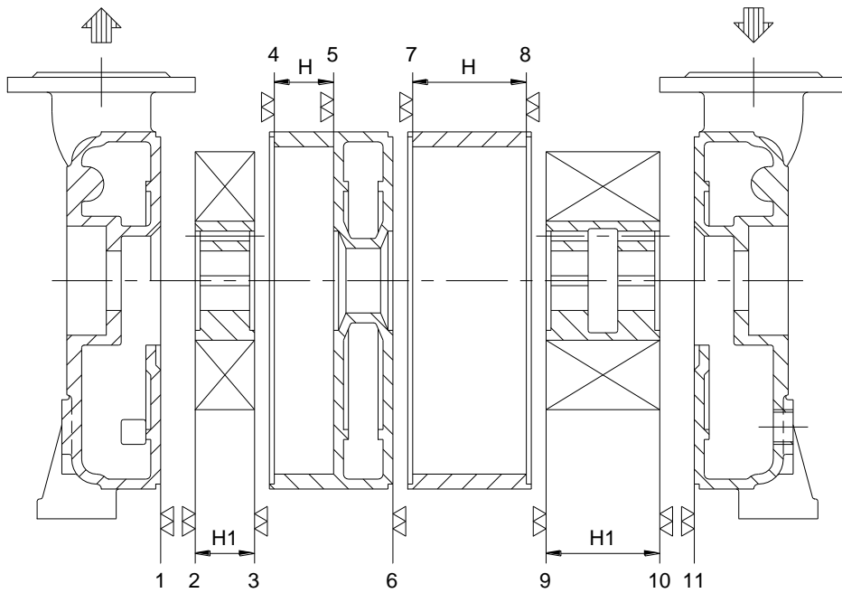
Fig. 14 TRHE 40 TRHB 50/GH - F - RA
