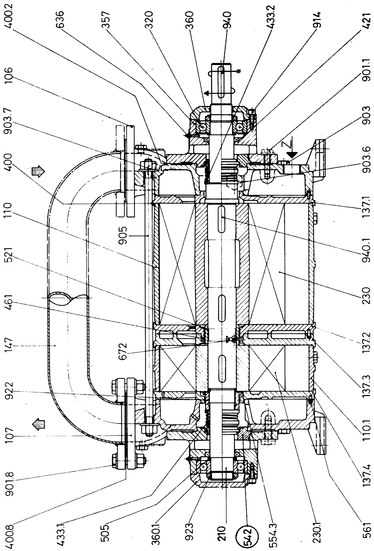
TRHC 80
