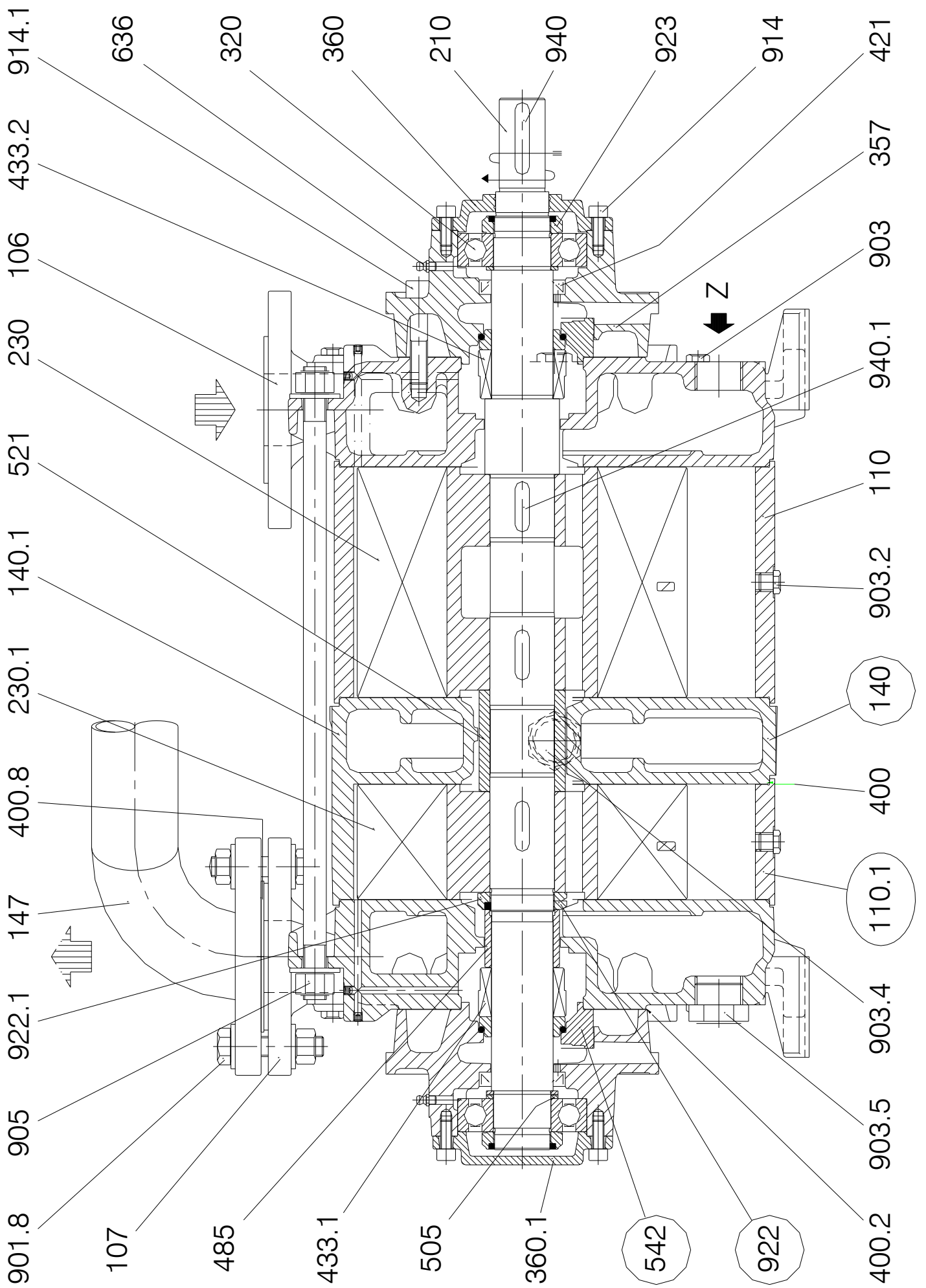
TRHB 50
