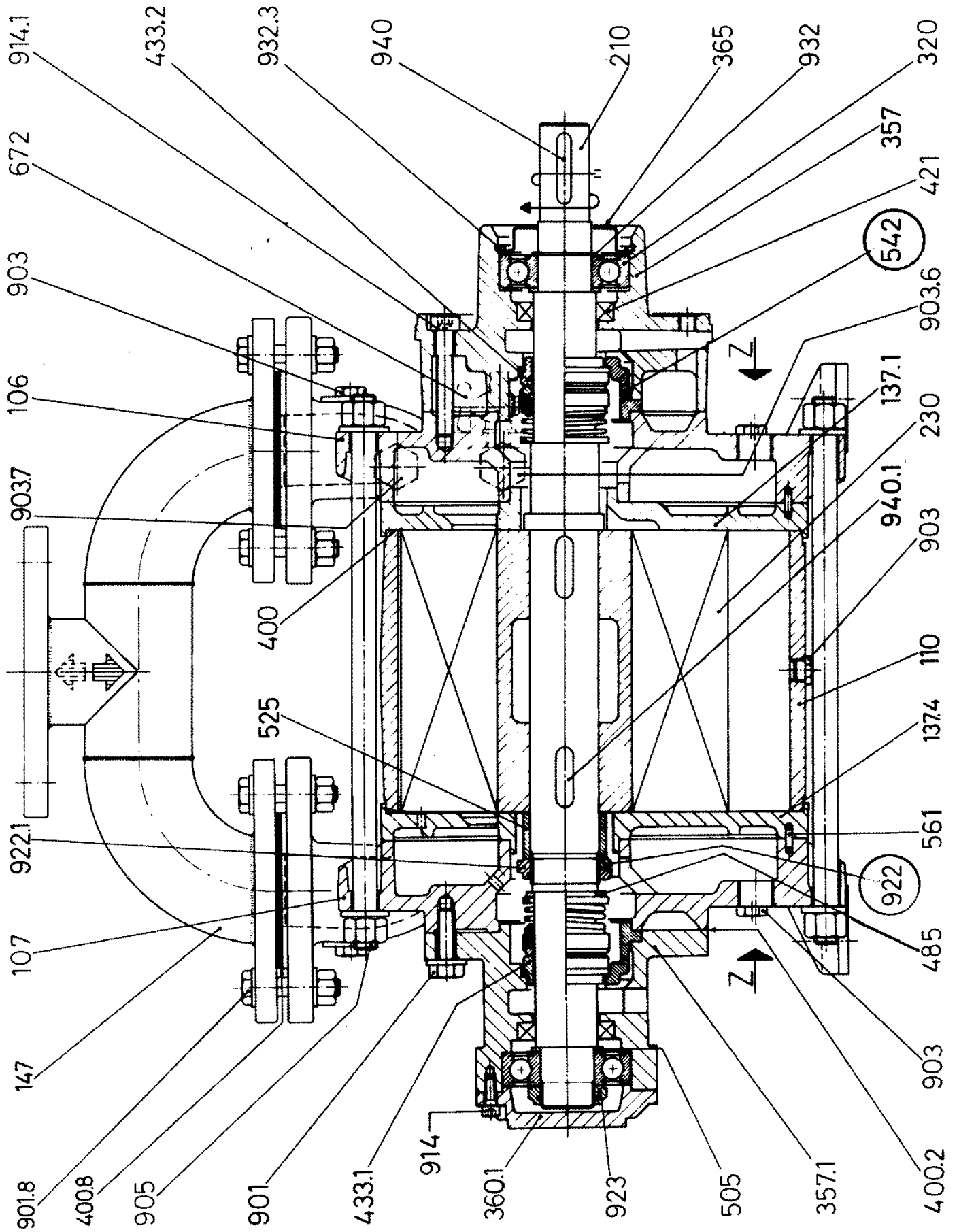
TRSC 50
