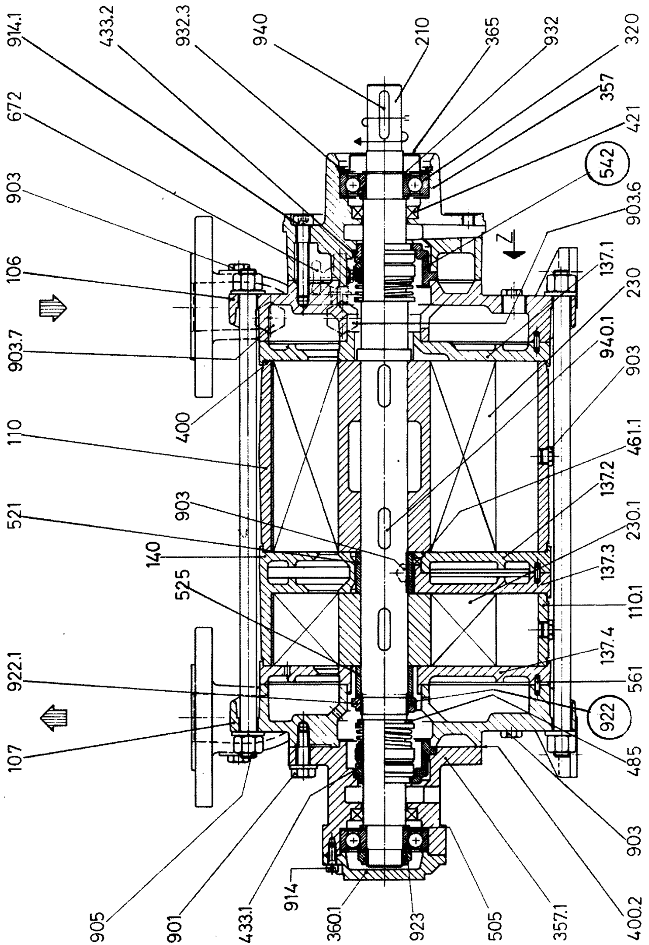
TRHC 40-110
