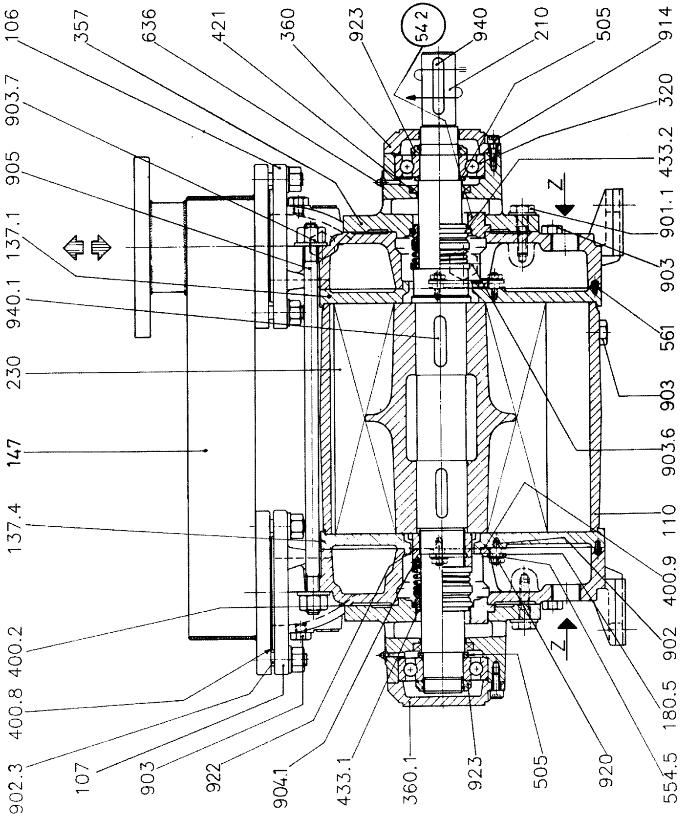
TRSC 100
