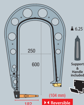
G5 8 bar/550 daN 022805
