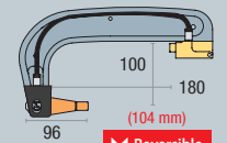
G1 8 bar/550 daN 022768
