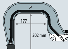
C3 8 bar/550 daN 021419
