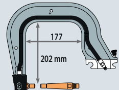
C8 8 bar/550 daN 021440
