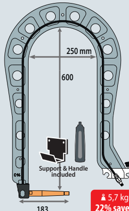
C14 8 bar/400 daN 023543
