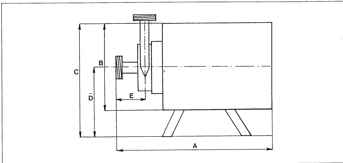
DIMENSIONI D'INGOMBRO IN mm DIMENSIONS
